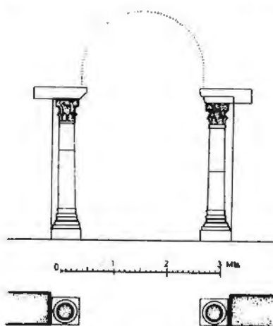
Fig. 1. Cornellà de Llobregat. Les columnes del segle X, planta i alçat, segons el Servei de Conservació de Monuments de la Diputació de Barcelona.
